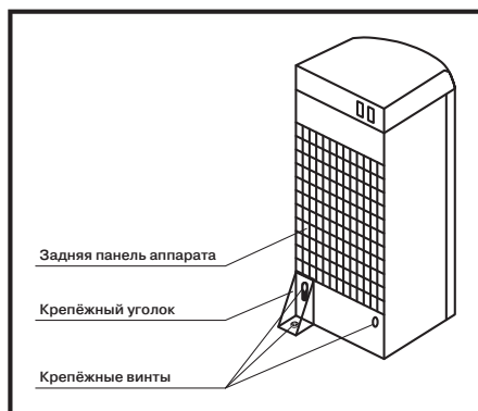
Рис. 2. Фиксация аппарата
