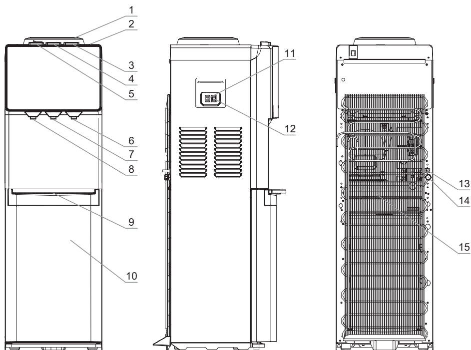
Рис. 1. Схема аппарата V400BS
