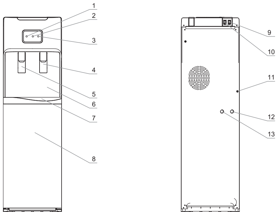
Мал. 1. Схема апарату V115AE
